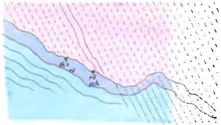
Fig. 6. Überspringen der Gneisschieferung auf den Kalk am Meltenberg (obere Contactlinie)
